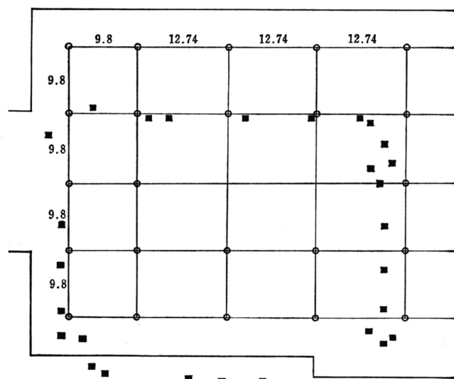
講堂基壇上面及び周辺の柱穴
