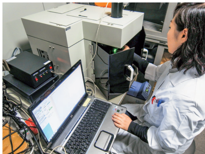
保存修復科学研究室：ガラス遺物のラマン分光分析 Conservation Science Section: Raman spectroscopy of ancient glass beads
