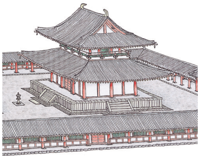
山田寺金堂・東回廊 復原図
